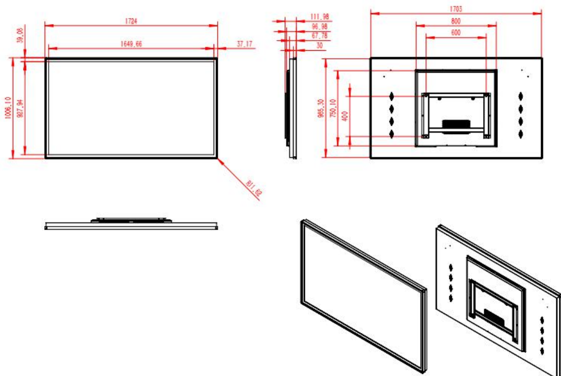
结构图
