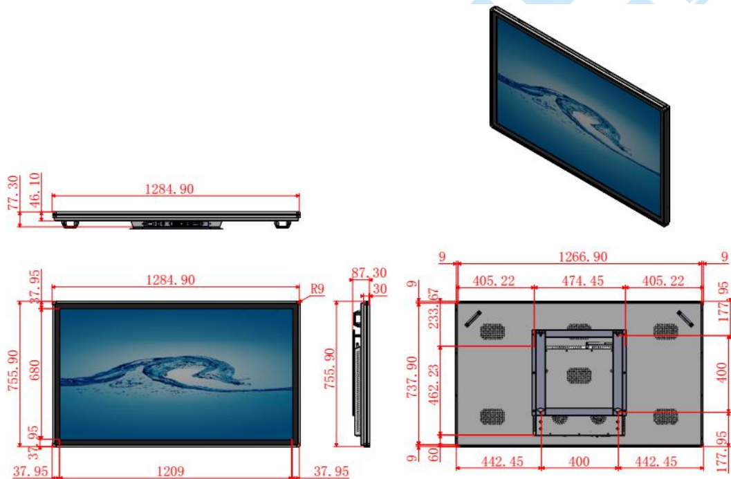
结构图
