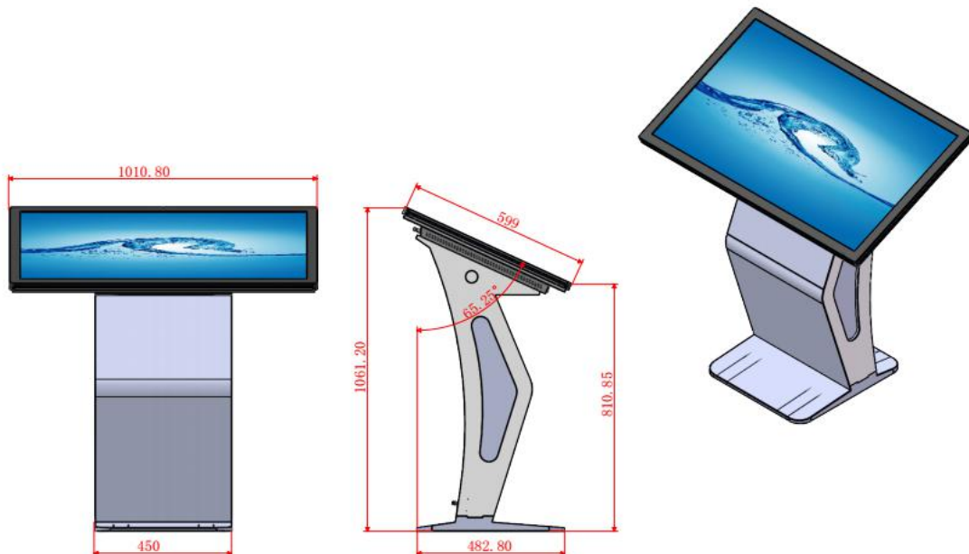
结构图
