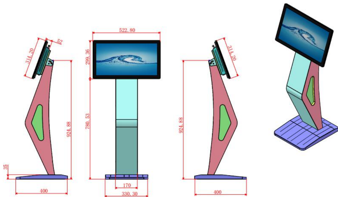
结构图
